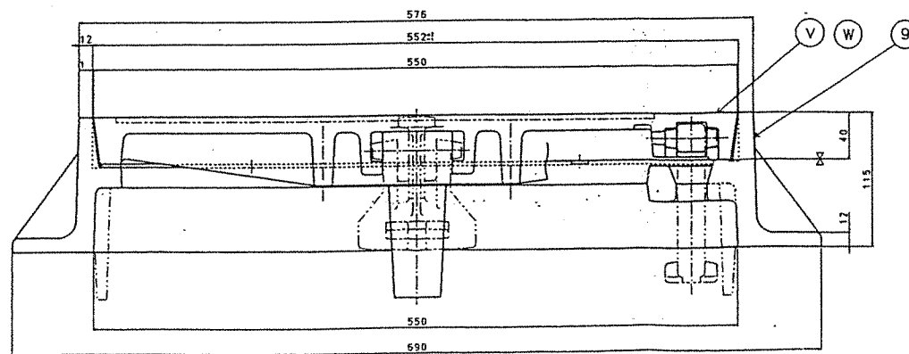
A - A 断面図
