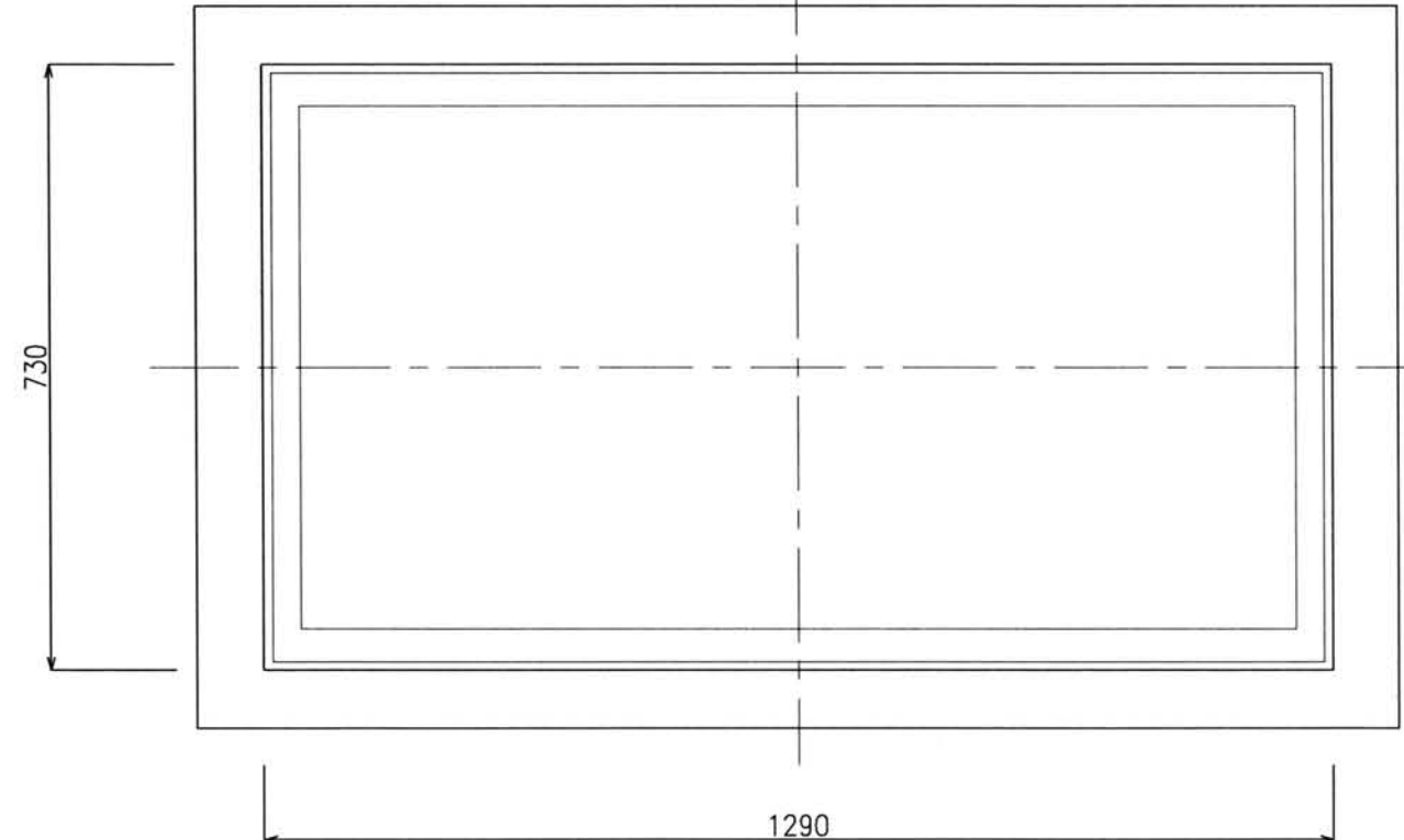
イ部 拡大図 1/2
