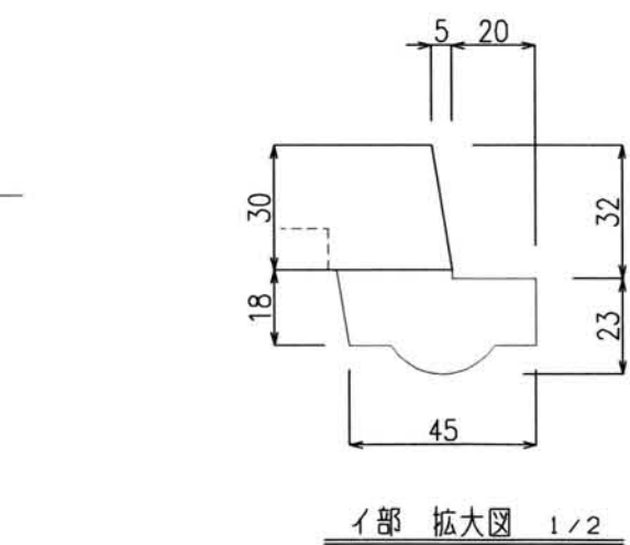
イ部 拡大図 1/2
